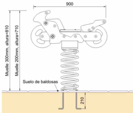
INSTALACIÓN SOBRE BALDOSAS
