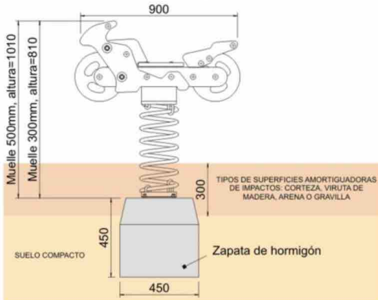
INSTALACIÓN EN SUELO DE ARENA
