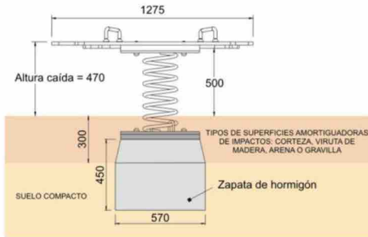
INSTALACIÓN EN SUELO DE ARENA
