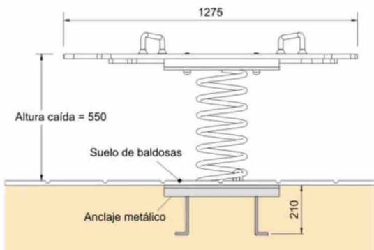
INSTALACIÓN SOBRE BALDOSAS
