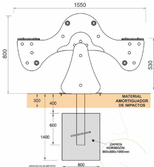
INSTALACIÓN EN SUELO DE ARENA
