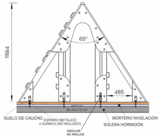
INSTALACIÓN EN SUELO DE HORMIGÓN
