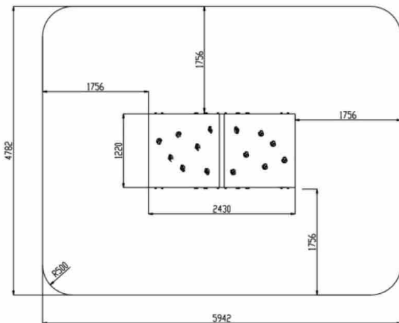
INSTALACIÓN EN SUELO DE TIERRA
