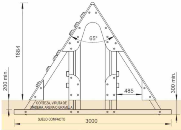
INSTALACIÓN EN SUELO DE TIERRA
